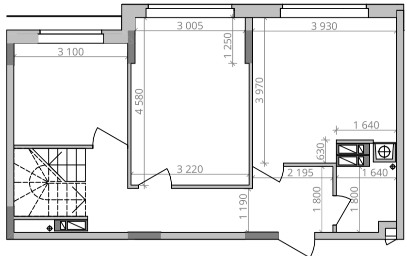
Габарити приміщень. 9 поверх. М 1:100
