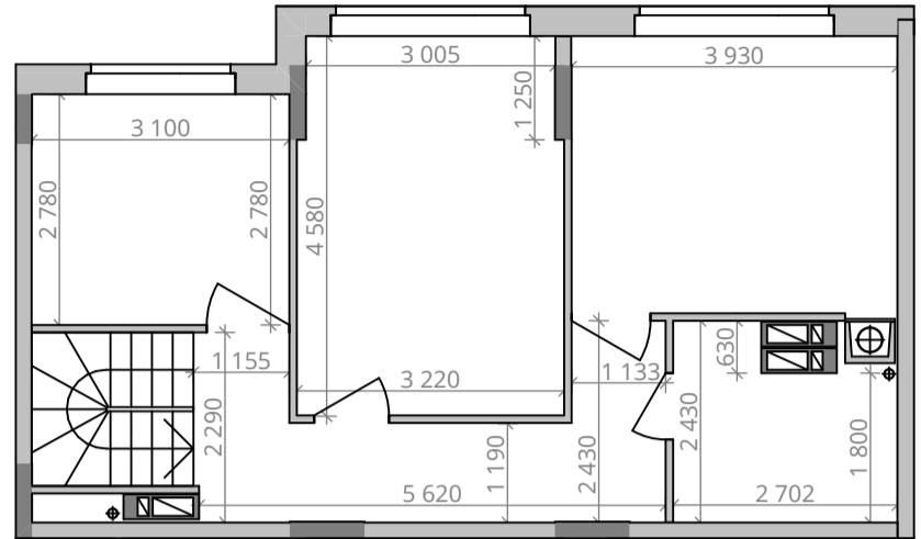
Габарити приміщень. 10 поверх. М 1:100
