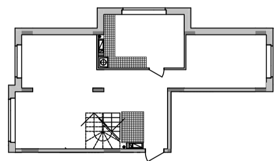
Схема перепланування. 9 поверх. М 1:200
