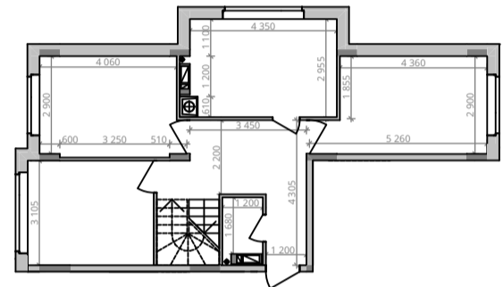
Габарити приміщень. 9 поверх. М 1:200
