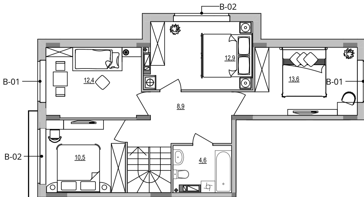
План квартири. 10 поверх. М 1:100
