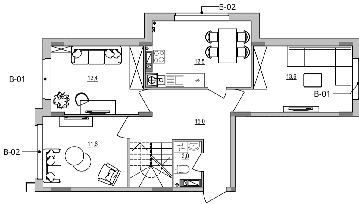
План квартири. 9 поверх. М 1:100
