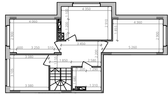
Габарити приміщень. 10 поверх. М 1:200
