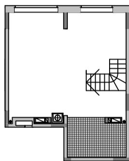
Схема перепланування. 10 поверх. М 1:200
