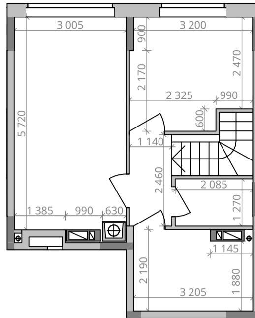
Габарити приміщень. 9 поверх. М 1:100
