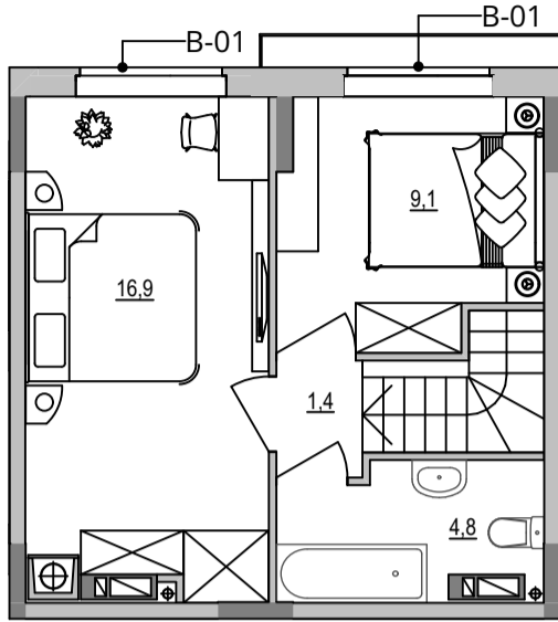
План квартири. 10 поверх. М 1:100
