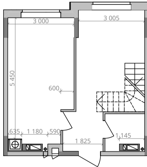
Габарити приміщень. 9 поверх. М 1:100
