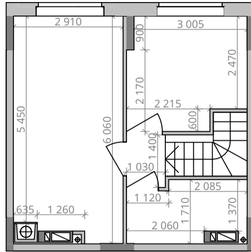
Габарити приміщень. 10 поверх. М 1:100
