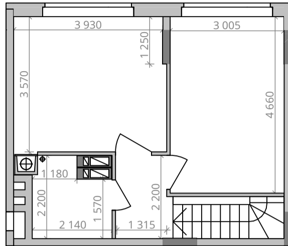
Габарити приміщень. 10 поверх. М 1:100
