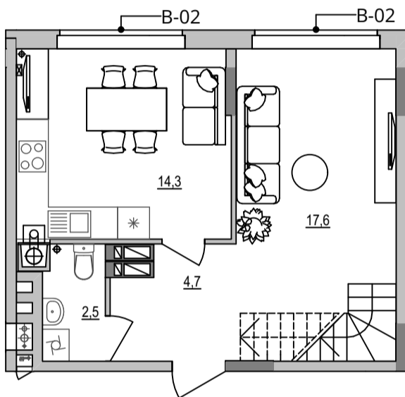
План квартири. 9 поверх. М 1:100
