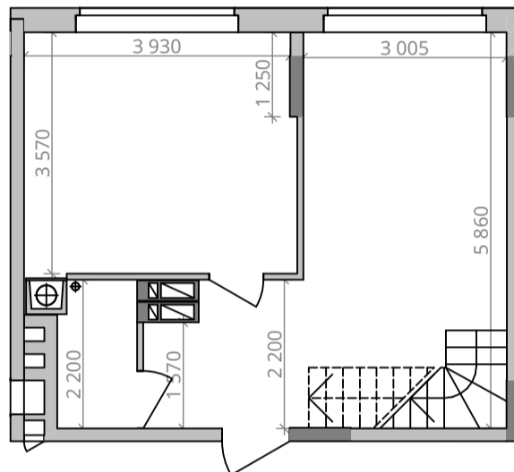
Габарити приміщень. 9 поверх. М 1:100
