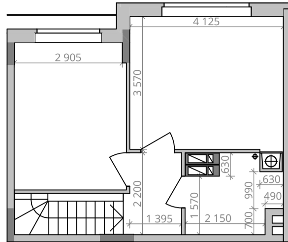
Габарити приміщень. 10 поверх. М 1:100
