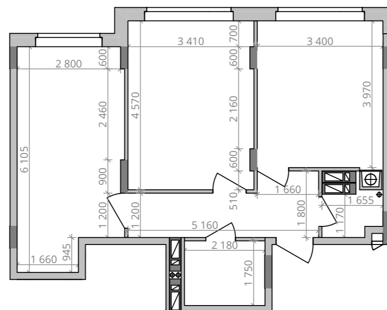
Габарити приміщень. М 1:100
