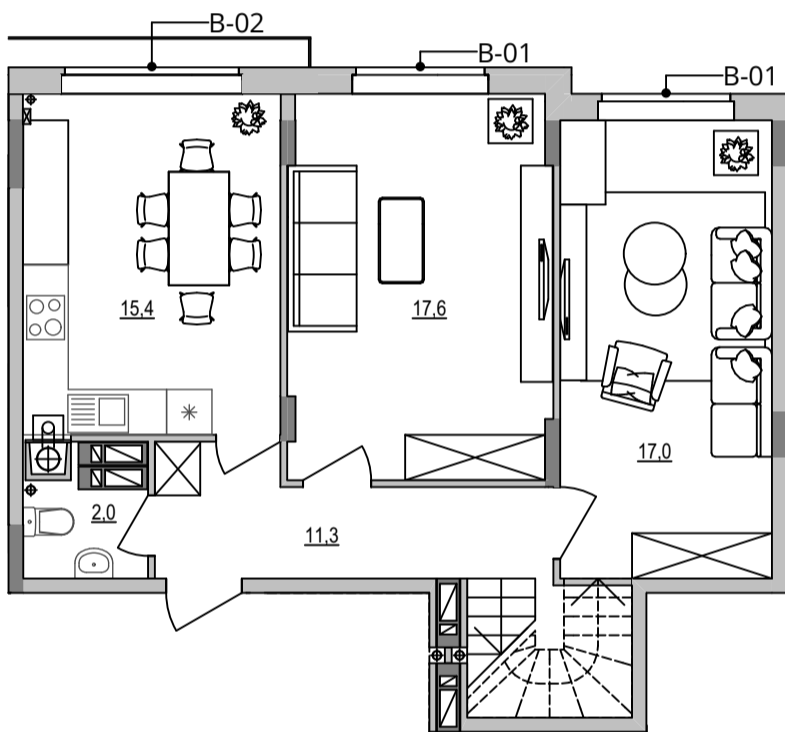
План квартири. 9 поверх. М 1:100
