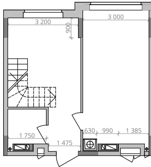
Схема перепланування. 9 поверх. М 1:200
