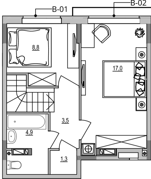
План квартири. 10 поверх. М 1:100
