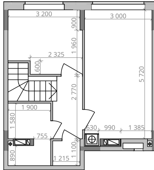
Габарити приміщень. 10 поверх. М 1:100
