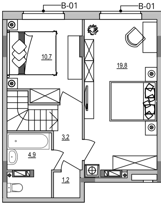
План квартири. 10 поверх. М 1:100
