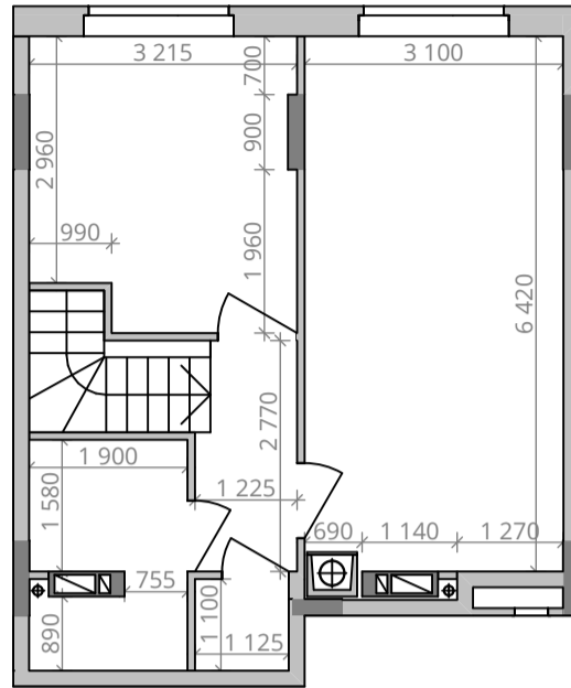
Габарити приміщень. 9 поверх. М 1:100
