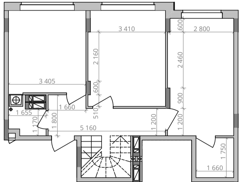
Схема перепланування. 9 поверх. М 1:200
