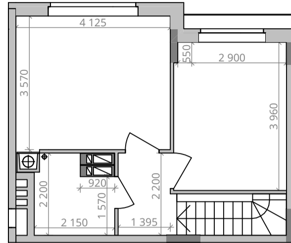
Габарити приміщень. 10 поверх. М 1:100
