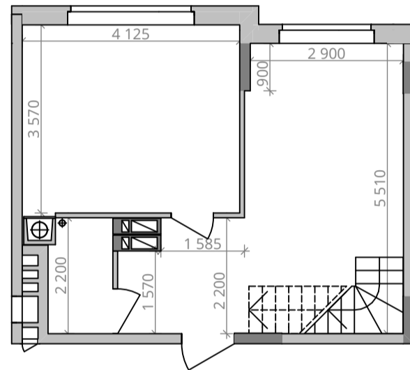
Габарити приміщень. 9 поверх. М 1:100
