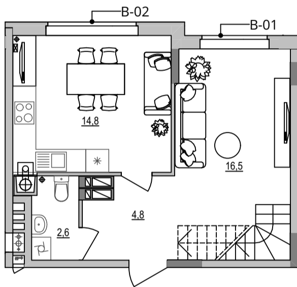
План квартири. 9 поверх. М 1:100
