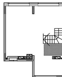
Схема перепланування. 9 поверх. М 1:200
