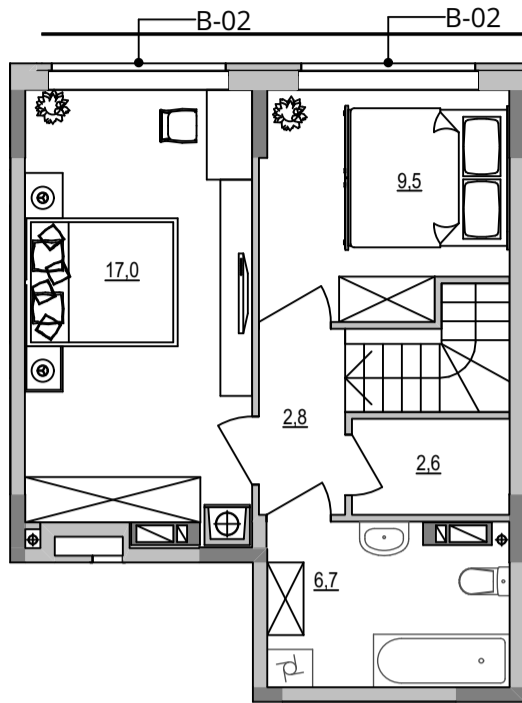
План квартири. 10 поверх. М 1:100
