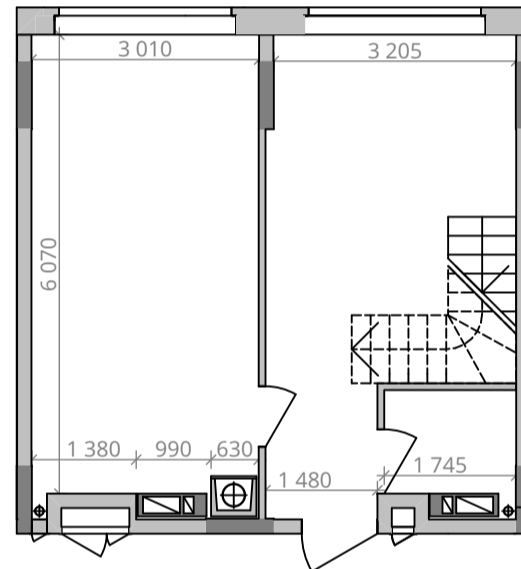
Схема перепланування. 9 поверх. М 1:200
