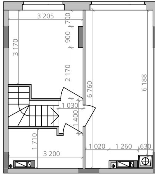
Габарити приміщень. 10 поверх. М 1:100
